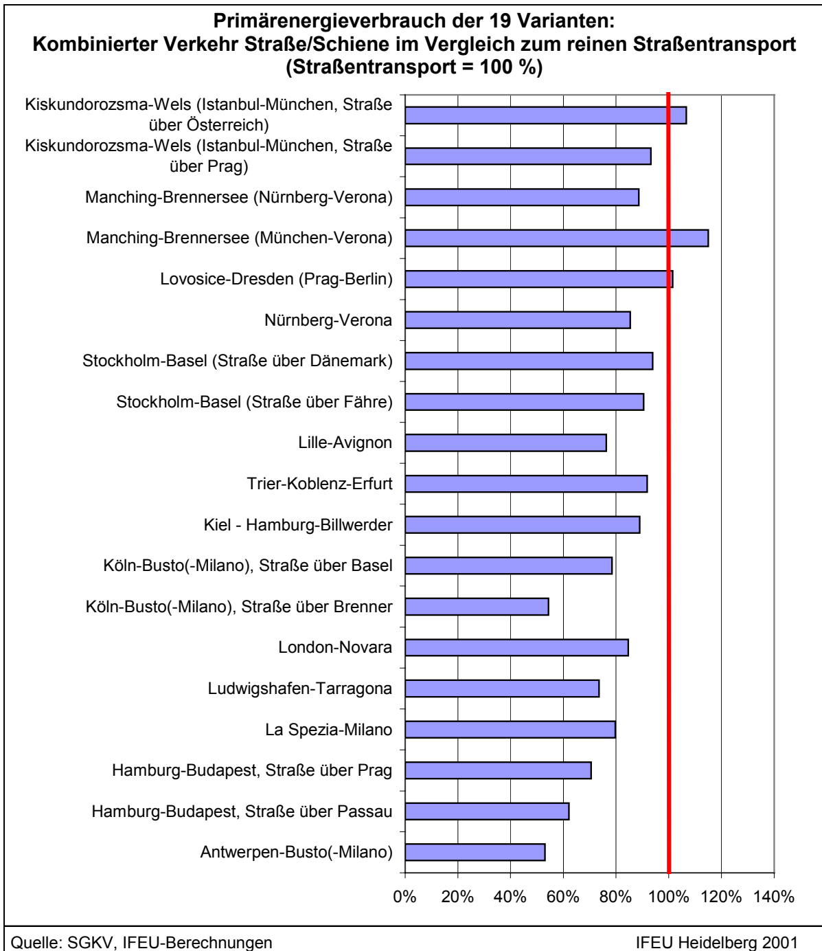
Abbildung 4 Primärenergieverbrauch der 19 Varianten: Kombiniertes Verkehr Straße/Schiene im Vergleich zum reinen Straßentransport
